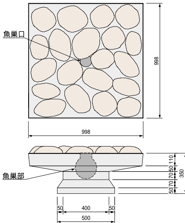
大型谷積みジャカゴブロックの形状・寸法
